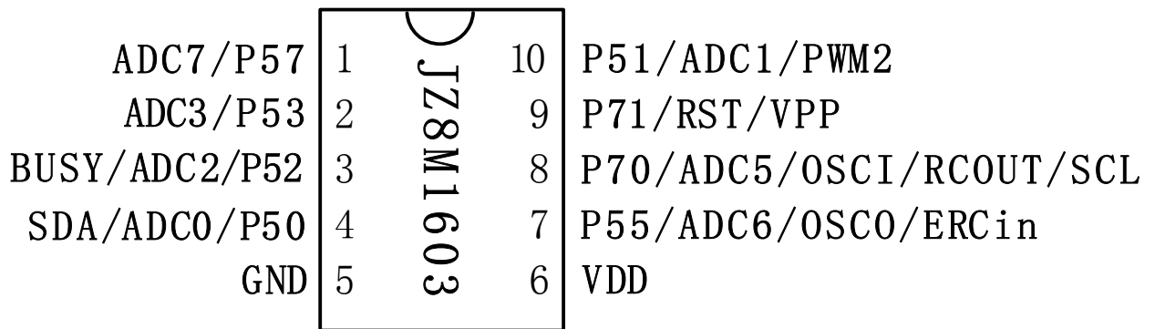
JZ8M1603-10PIN 脚位图
