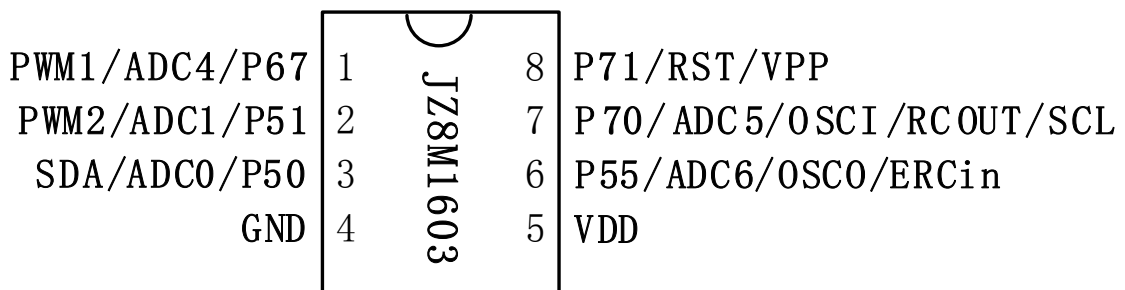
JZ8M1603-8PIN 脚位图
