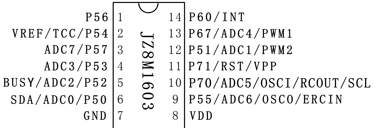
JZ8M1603-14PIN 脚位图
