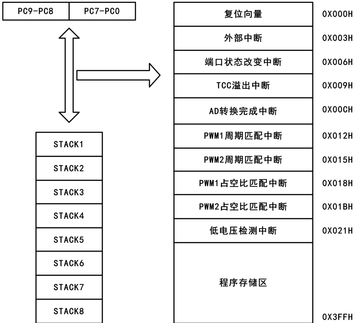
程序存储器区结构图
