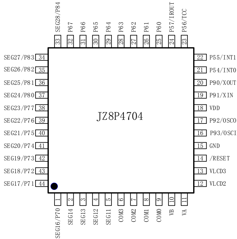
JZ8P4704-44PIN 脚位图
