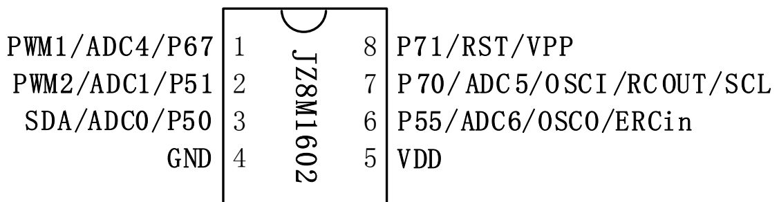
JZ8M1602-8PIN 脚位图
