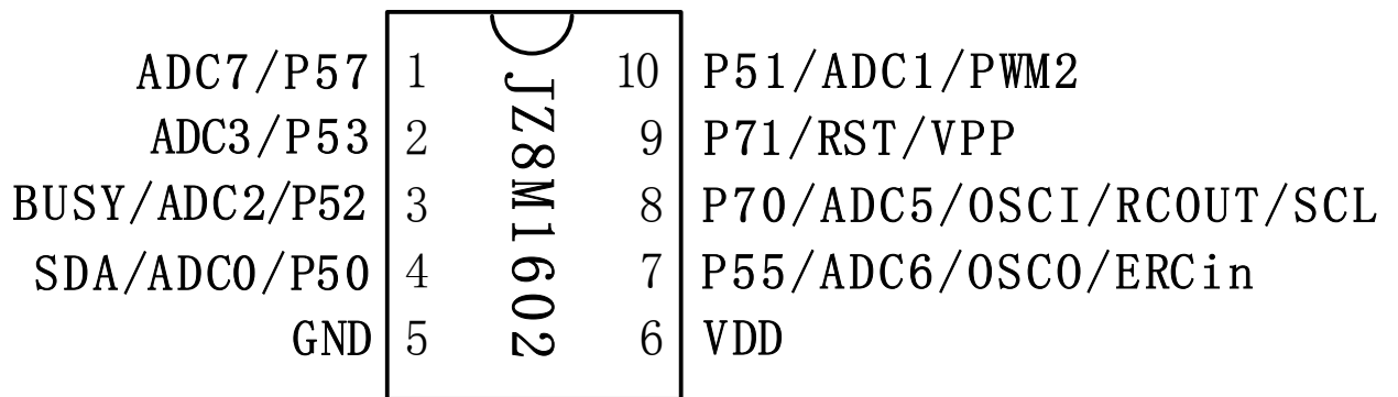
JZ8M1602-10PIN 脚位图
