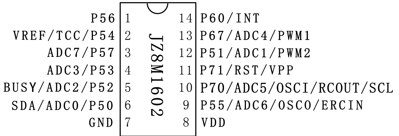
JZ8M1602-14PIN 脚位图
