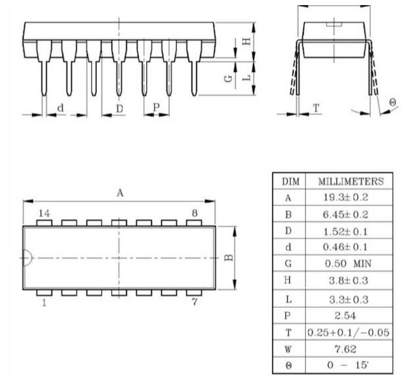
DIP14 封装尺寸
